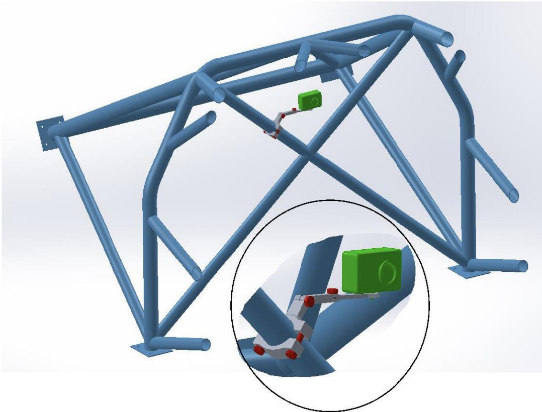
Cámara tipo caja en la cruz del arco principal
